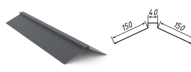
Планка ендовы нижняя
