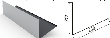
Планка верхнего примыкания к трубе
