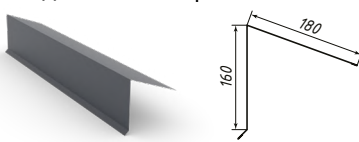
Планка верхнего примыкания к трубе
