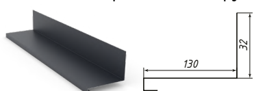
Планка нижнего примыкания к трубе
